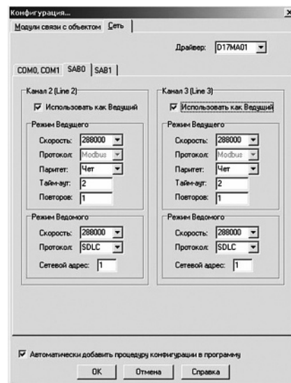
Рис. 2. Конфигуратор информационных каналов контроллера
