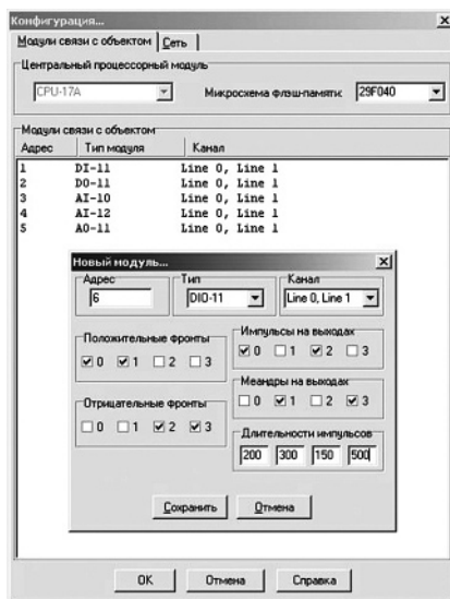
Рис. 1. Конфигуратор модулей удаленной связи с объектом серии DCS-2000
