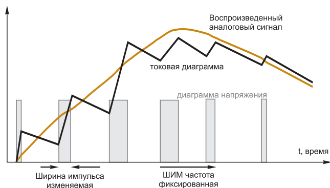
Рис. 2. Воспроизведение аналогового сигнала с помощью широтно-импульсной модуляции (ШИМ) Показано воспроизведение хода аналогового сигнала через относительную длительность прямоугольного импульса внутри заданного такта (периода), который должен быть тем короче, чем динамичнее процесс. ШИМ применяется в электротехнике, например для дискретного управления пропорциональными клапанами и электромагнитами. При прохождении каждого импульса в катушке возникает средний ток, который подается только во временной интервал, равный длине импульса/паузы. Преимущества метода заключается в значительном уменьшении рассеиваемой мощности дискретного шим-модуля (почти не нагревается) по сравнению с аналоговым модулем (нагревается)
