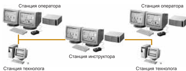
Структурная схема тренажера ХВО
