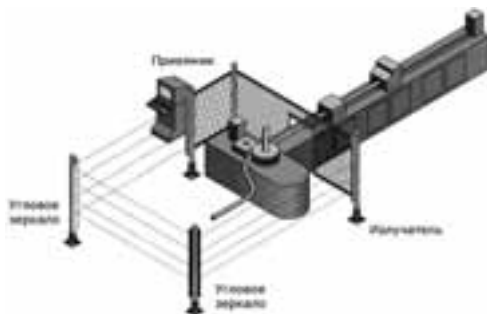
Рис. 2. Контроль периметра машины
