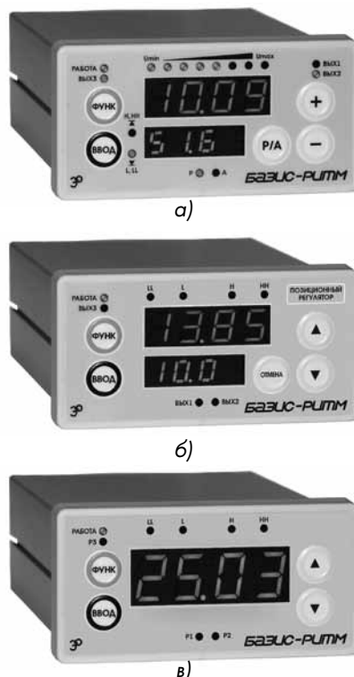
Рис. 1. Исполнения контроллера БАЗИС-РИТМ: а) БАЗИС-РИТМ.ТОК/РИМ/ШИМ; б) БАЗИС-РИТМ.П (с двумя индикаторами); в) БАЗИС-РИТМ.И (с одним двухцветным индикатором)
