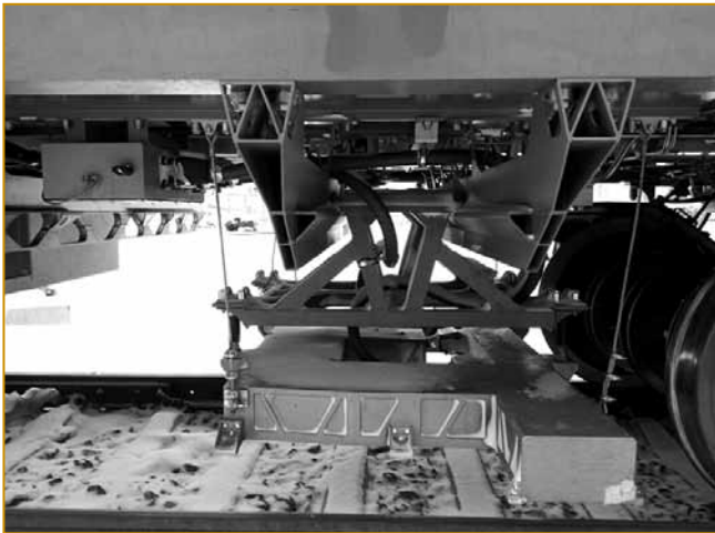
Рис. 3. Система контроля состояния геометрии пути и рельсов
