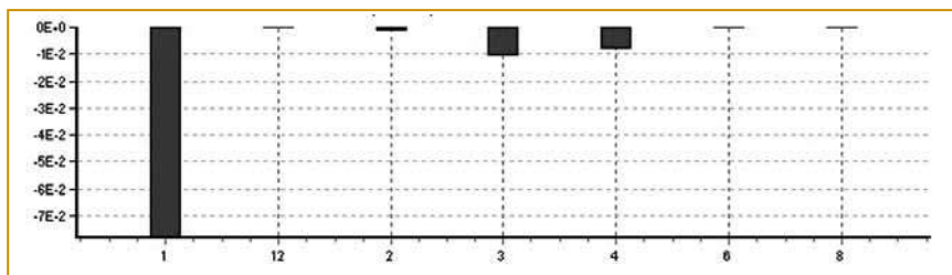
Рис. 6. Диаграмма отрицательных вкладов отдельных событий в вероятность отказа электрогенератора
