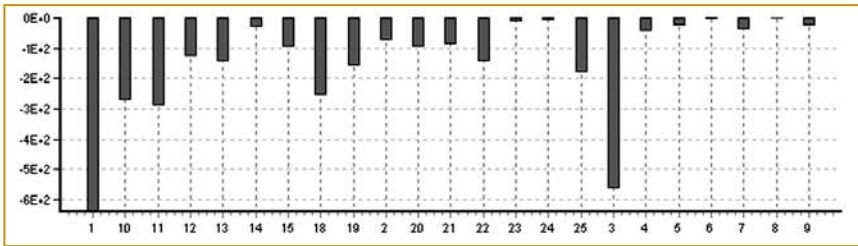
Рис. 3. Диаграмма распределения рисков по событиям дерева событий
