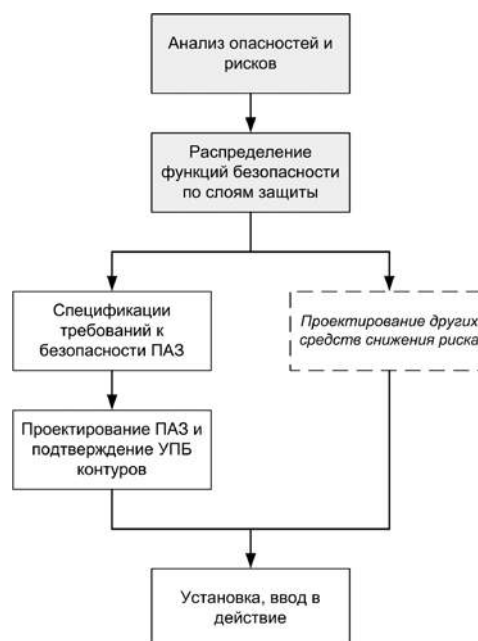
Рис. 1. Фрагмент жизненного цикла функциональной безопасности системы ПАЗ
