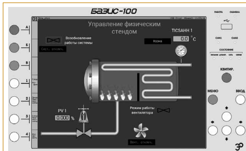
Рис. 3. Пользовательский интерфейс панели оператора
