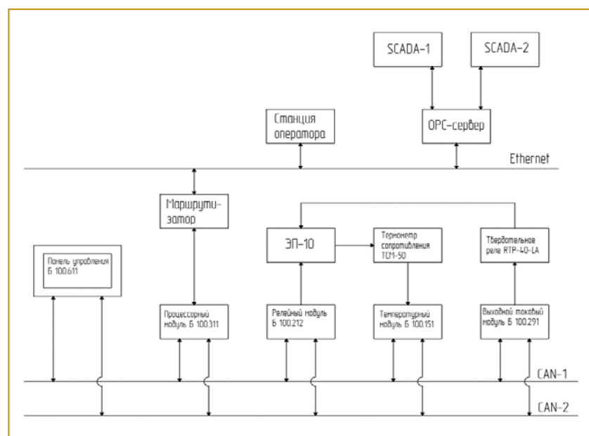
Рис. 2. Структурная схема лабораторного стенда
